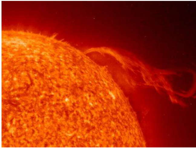
Протуберанец
