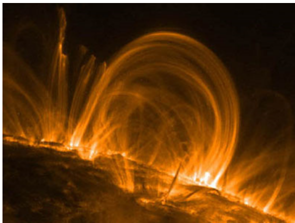
Корональные арки
